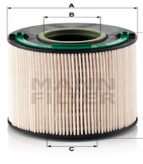
Fuel Filter PU 1040 x EM-20048
